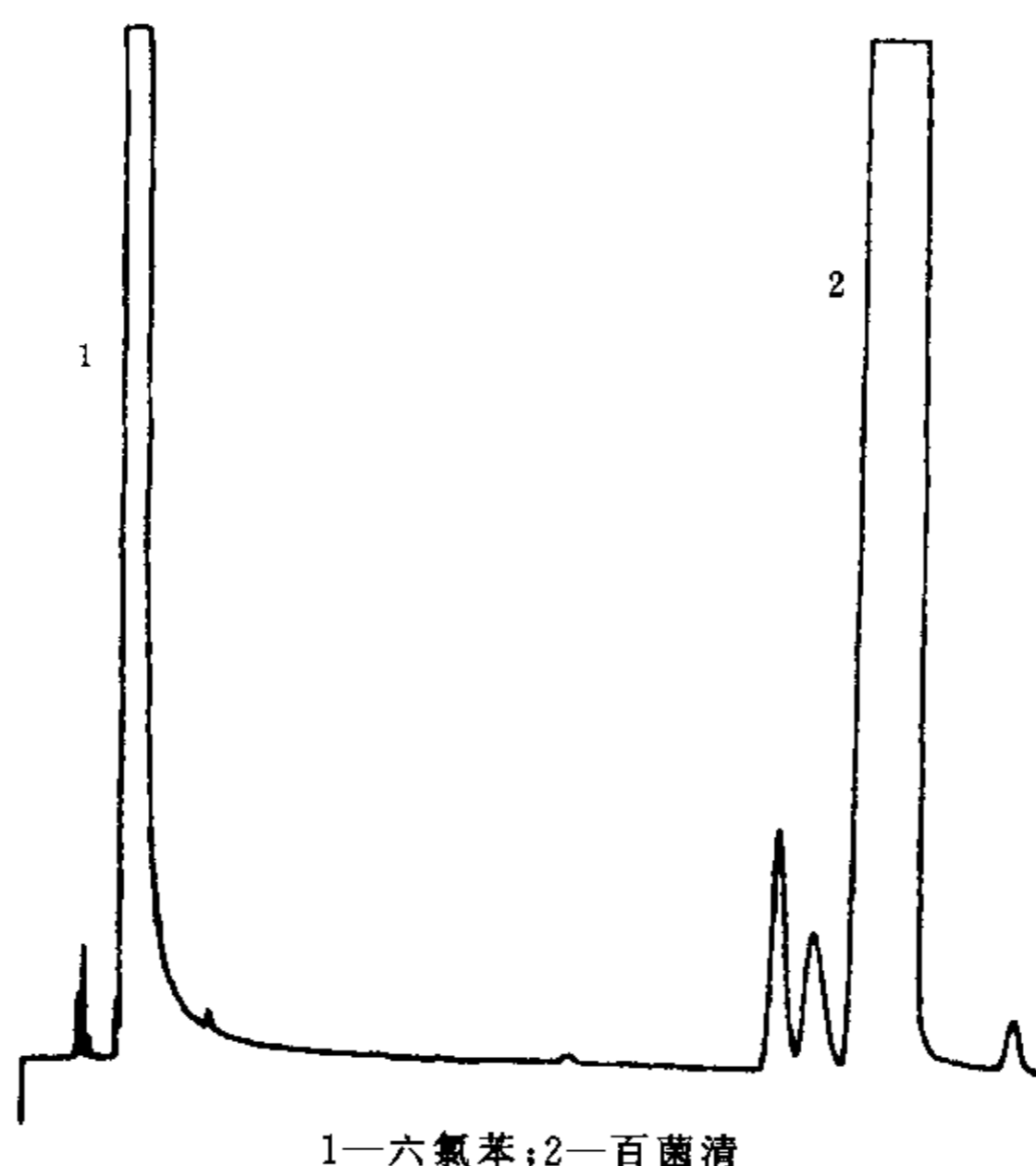
图 A1 百菌清粉剂试样的色谱图
