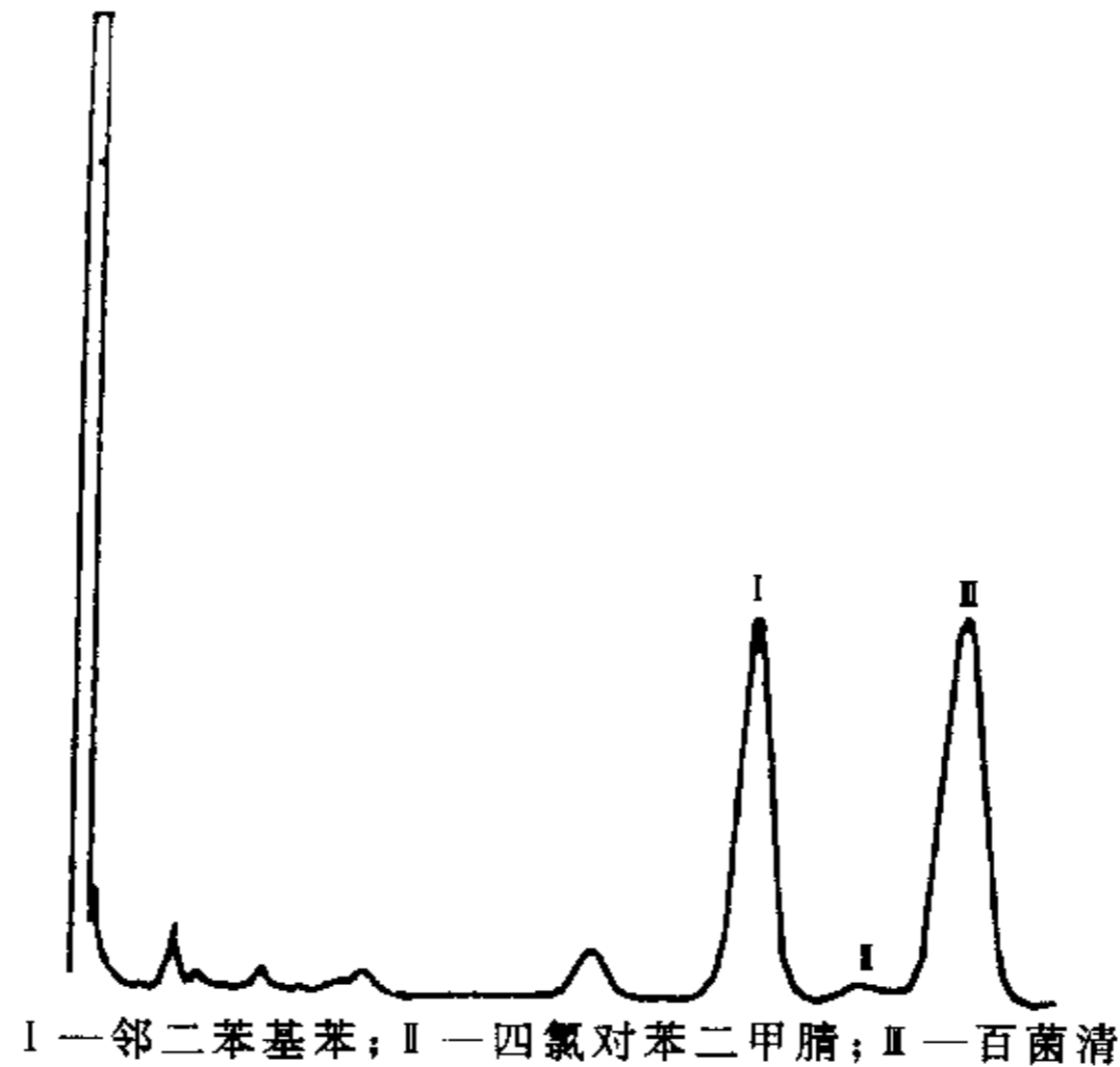
图 1 百菌清可湿性粉剂气相色谱图
